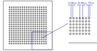
12 x 12 mm kare % 21 boşluklu
