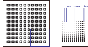
8 x 8 mm kare % 22 boşluklu
